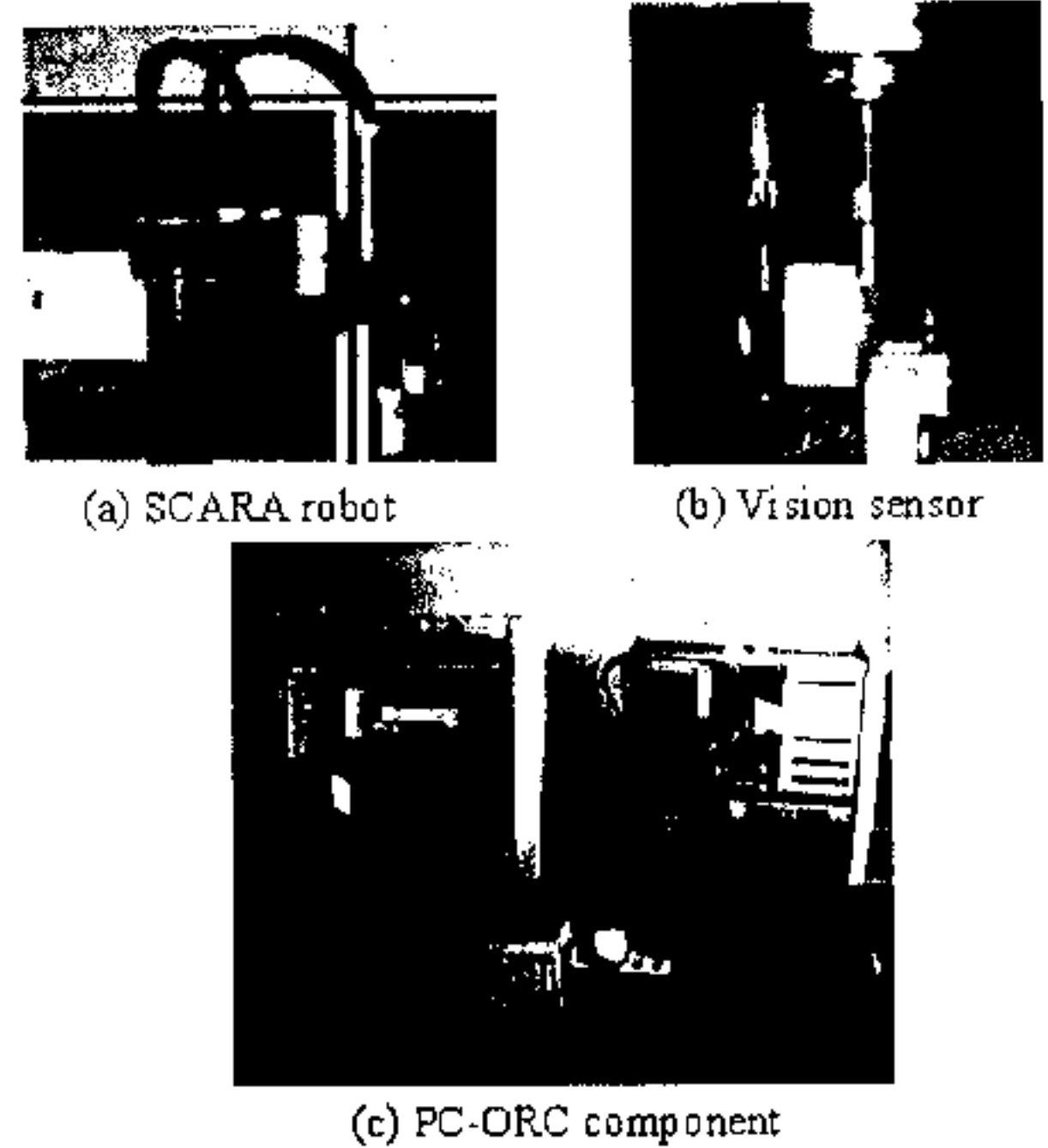
그림 9. 스카라로봇에 적용된 PC-ORC의 실험장비. Fig. 9. An experimental setup of the PC ORC applied to the SCARA robot.
