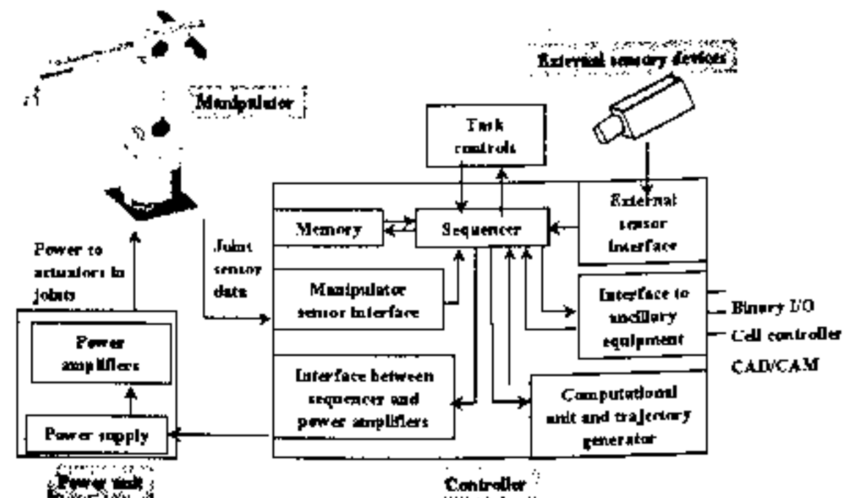
그림 2. 일반적인 산업용 로봇시스템의 구성요소 Fig. 2. Various elements of a general industrial robot.
