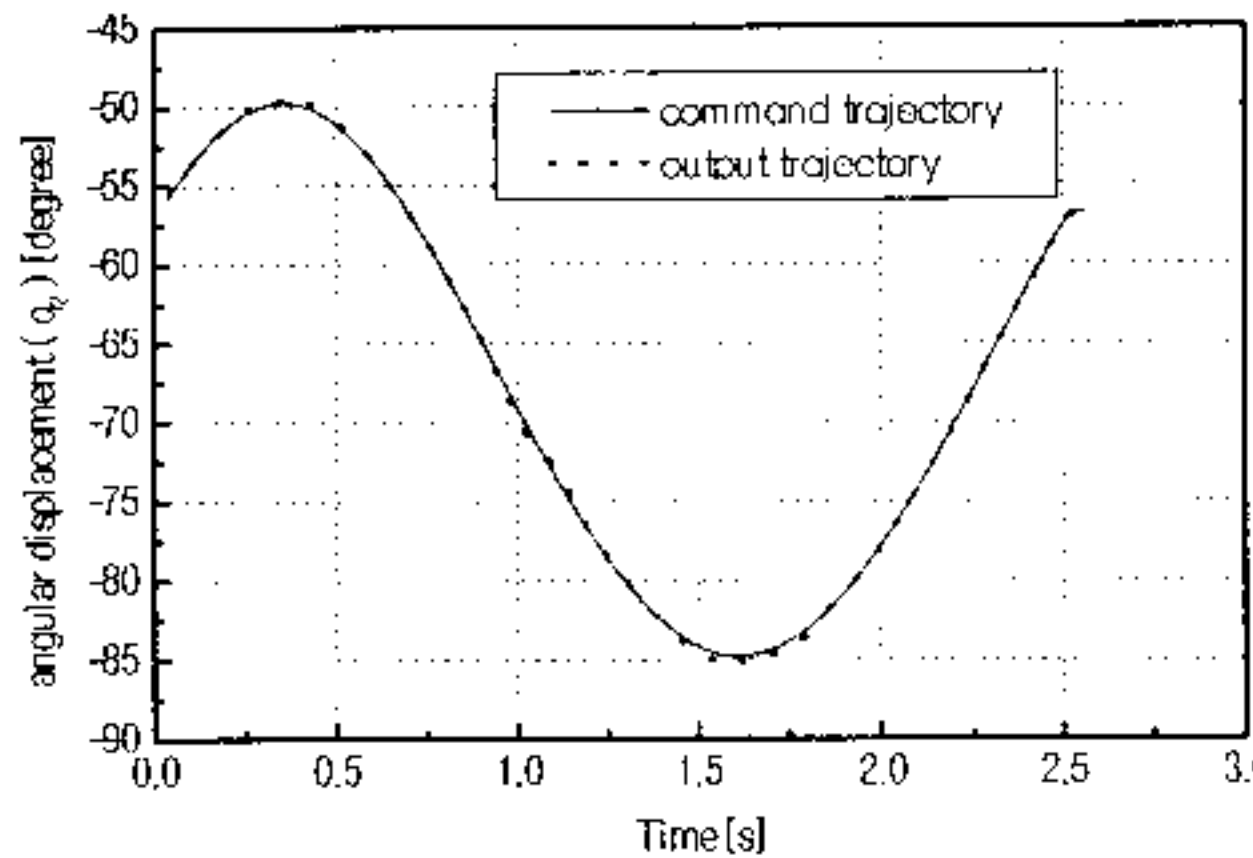
그림 14. 스카라로봇 제2축의 명령추종실험.
