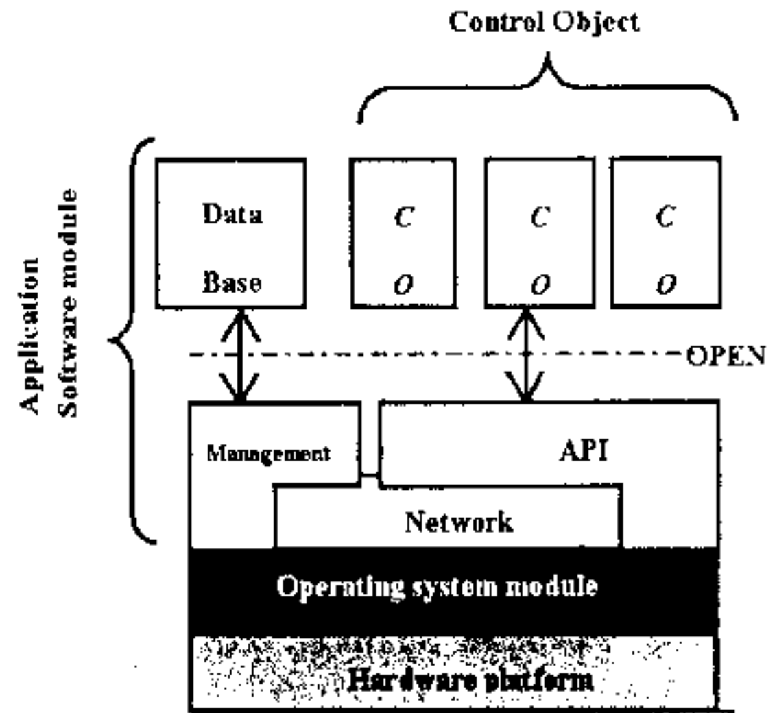
그림 1. 제안된 PC-ORC를 위한 표준기준모델.
